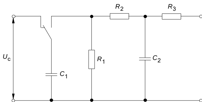
รูปที่ ณ.1 วงจรกำเนิดอิมพัลส์
