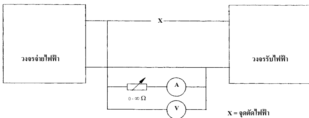
รูปที่ 1 วงจรทดสอบสำหรับภาวะผิดปกติ (ข้อ 2.3.7, ข้อ 4.3)
