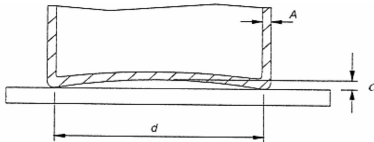
รูปที่ 103 ภาชนะสำหรับการทดสอบเตาแผ่นความร้อน (ข้อ 3.1.9.108)
