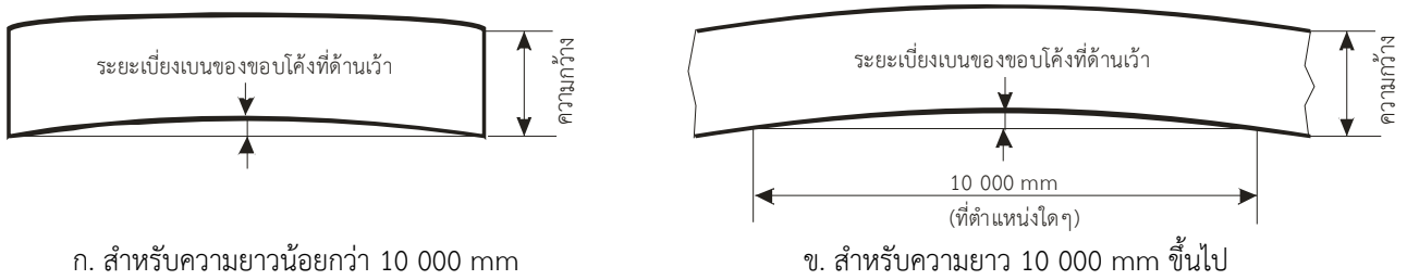
รูปที่ 2 การวัดระยะเบี่ยงเบนของขอบโค้งที่ด้านเว้าของเหล็กแผ่นหนา/แผ่นบางขอบตัด (ข้อ 6.5)
