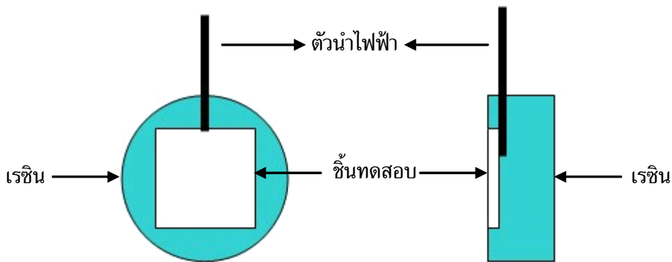
รูปที่ 1 แสดงการติดตัวนำไฟฟ้าและขั้วเรซินชั้นทดสอบ (ข้อ 9.6.3.2)
