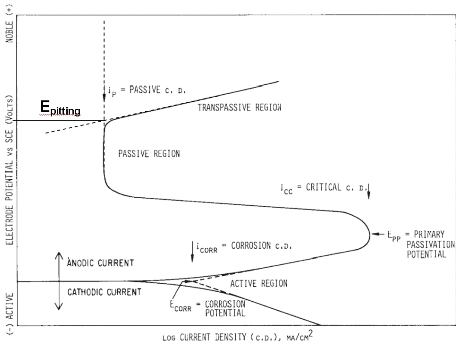
รูปที่ 3 กราฟแสดงเส้นโค้งโพลาริเซชัน(polarization curve) แสดงค่า i_{corr} , E_{corr} , E_{pitting} (ข้อ 9.6.4.5 (3) ข้อ 9.6.4.6 และข้อ 9.7.4.5(3))
