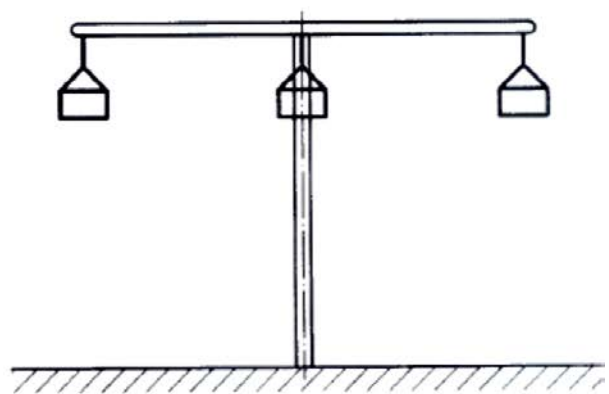
รูปที่ 3 ตัวอย่างผ้าหมุนแบบ C (ข้อ 2.5)
