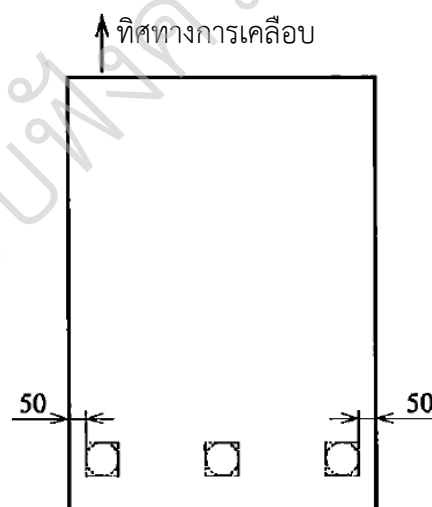
รูปที่ 2 ตำแหน่งขึ้นทดสอบมวลเคลือบ (กรณีทำโดยกรรมวิธีจุ่มร้อนแบบต่อเนื่อง)
