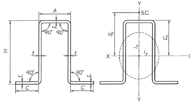
ตารางที่ ก.6 ขนาด ความหนา รูป และมวลต่อเมตรของเหล็กรูปหมวก (ข้อ ก.1)
